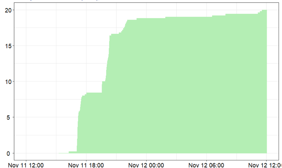
Figura 5. Precipitación horaria acumulada en la ciudad de Osorno el 11 de noviembre de 2022. Datos: DMC
