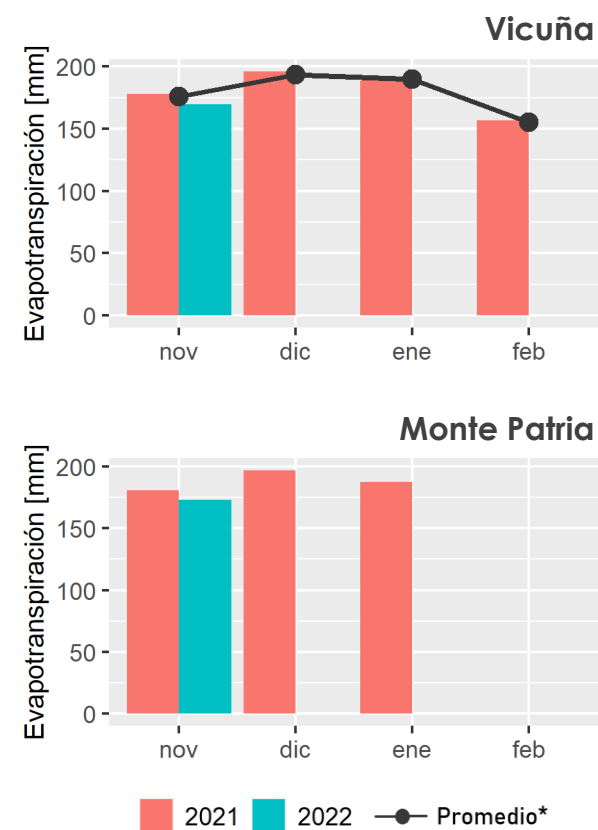
Figura 12. Evapotranspiración acumulada mensual para dos localidades del Norte Chico entre noviembre 2021 y febrero 2022, noviembre 2022 y promedio. Datos: DMC. *Promedio de Vicuña obtenido en 5 años de datos. Para Monte Patria no fue posible obtener el promedio.
